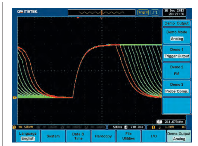
Рис. 10. Контроль демонстрационного ЧМ-сигнала
