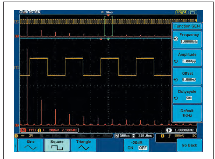
Рис. 15. Осциллограммы и спектр меандра в линейном масштабе
