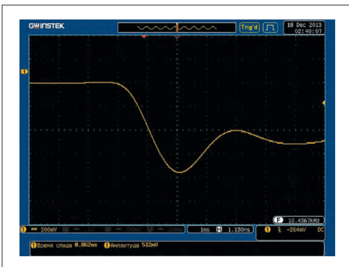
Рис. 5. Переходная характеристика аналоговых каналов
